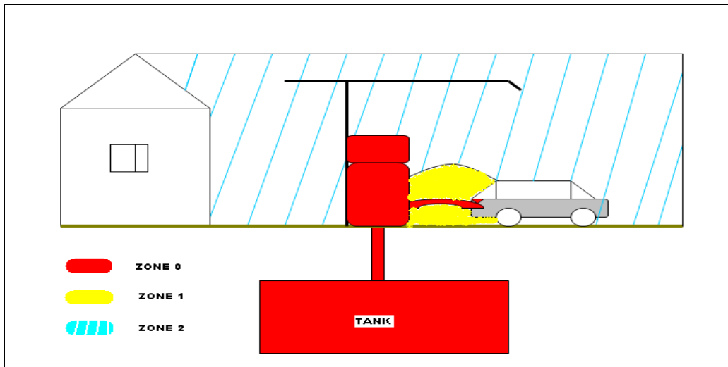
Şekil 1 Akaryakıt istasyonunda zone ayrımı
