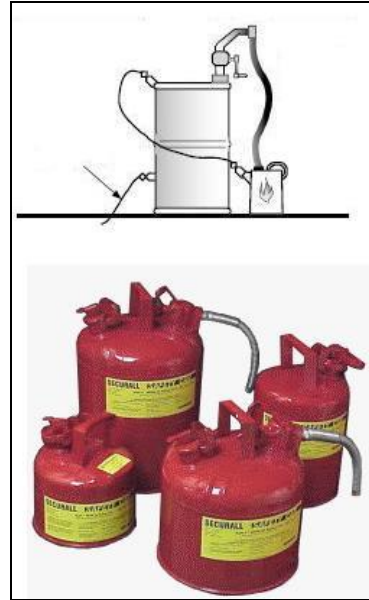
Resim 14 Kimyasalın varilden kapalı devre sistemle alınması ve taşındığı çelik bidonlar (Asecos)
